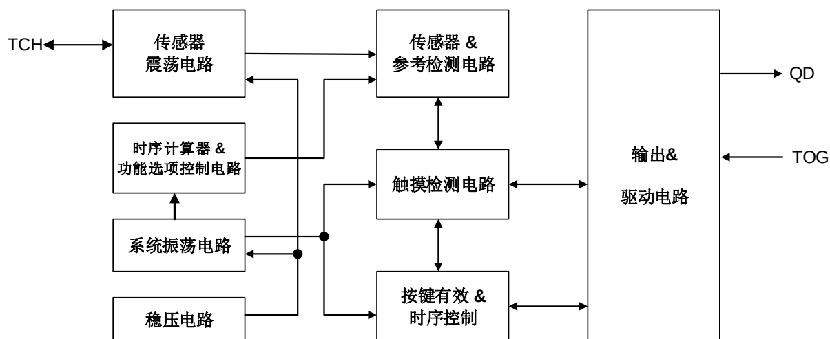
图 1 系统框图
