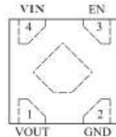
Package Type : DFN1*1-4L
